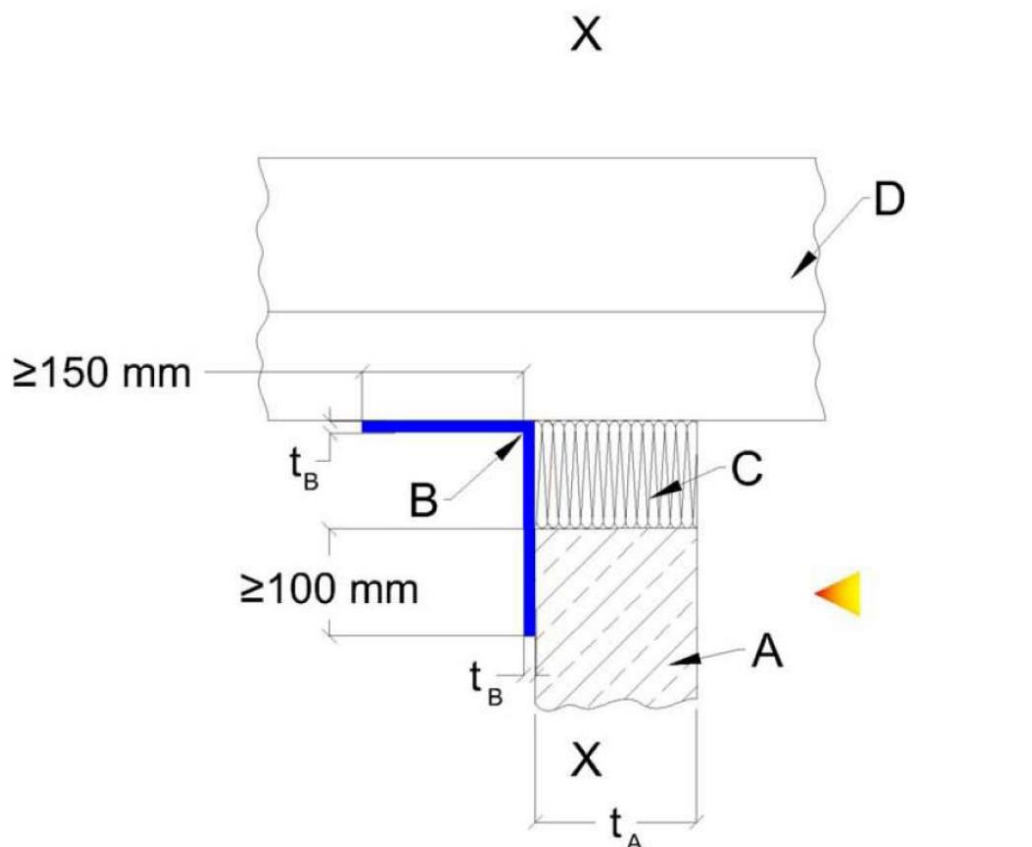
przekrój X-X
