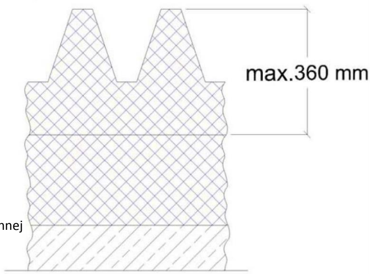
przekrój X-X
