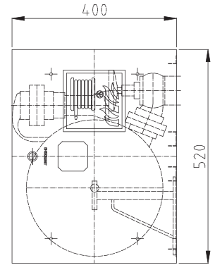
Wymiary hydrantu
