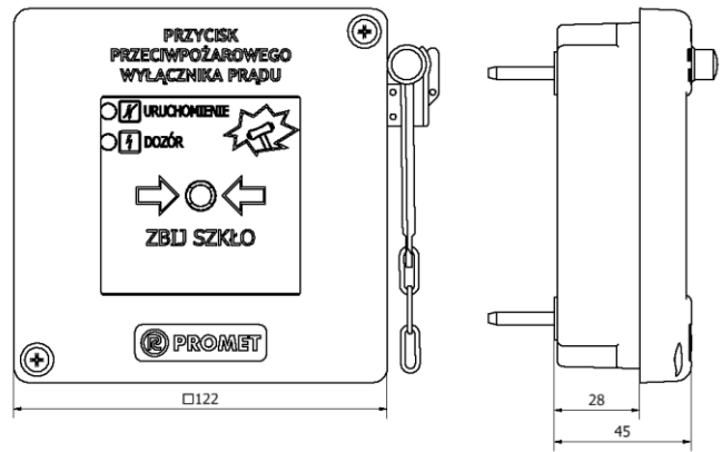
Rys. 2. Wymiary gabarytowe
